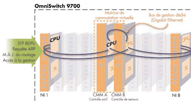
Principe de fonctionnement de l'intelligence distribuée
